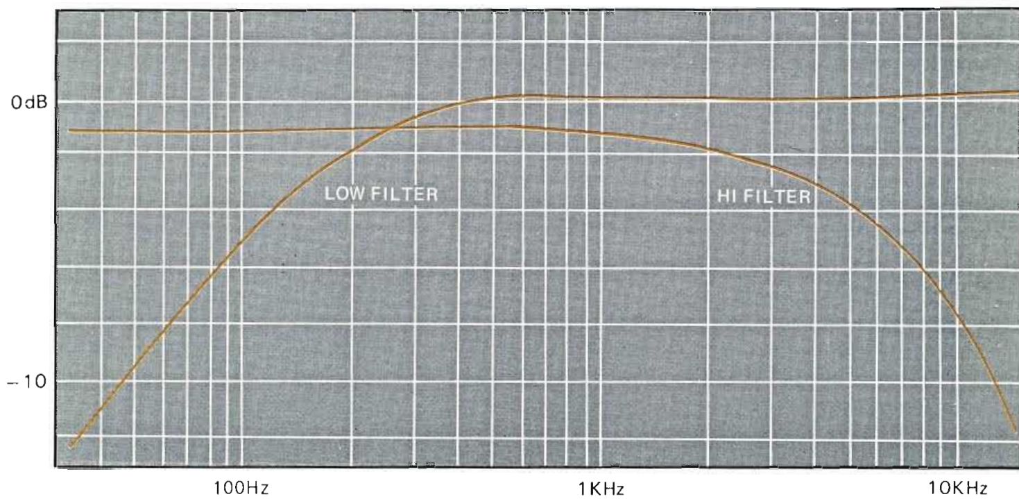
Figure 8. Caractéristiques des filtres passe-bas et passe-haut
