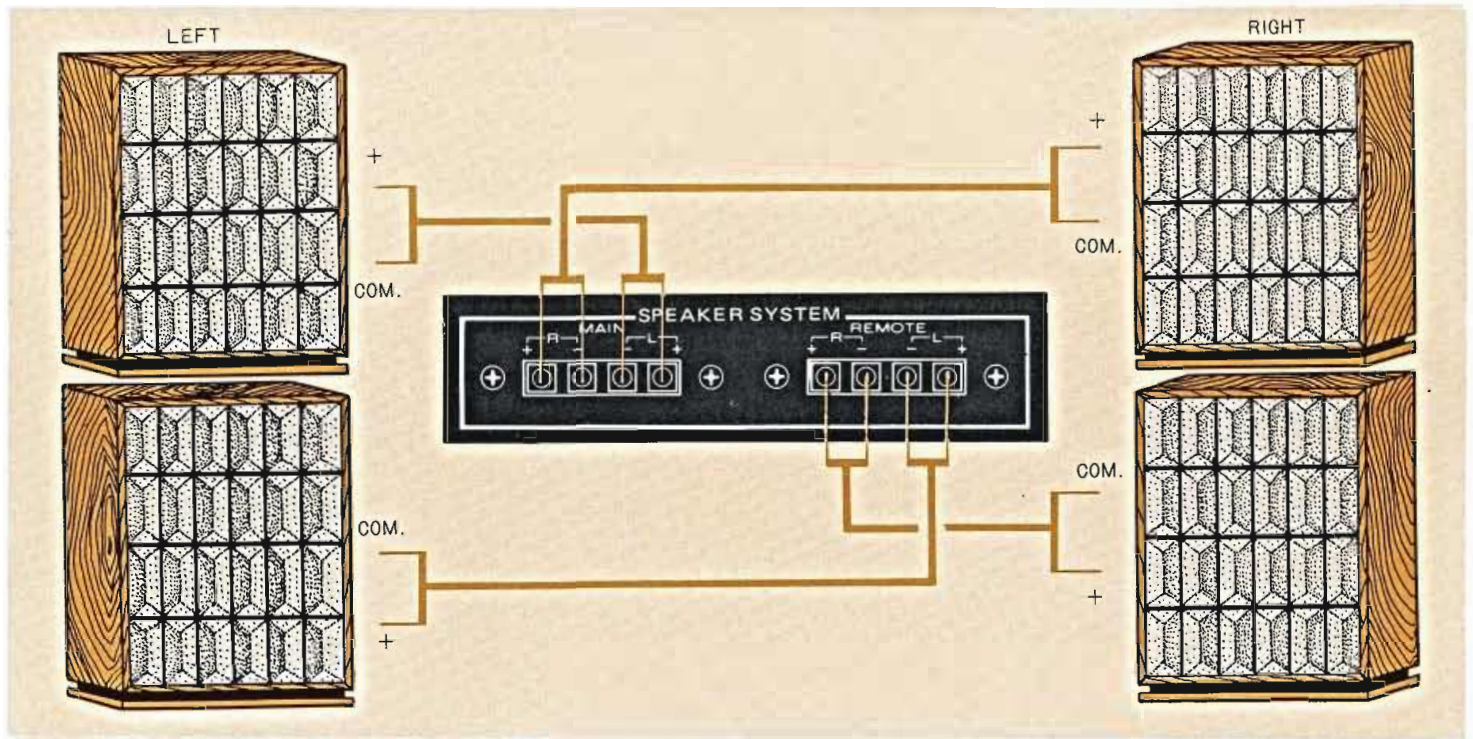
Figure 2. Raccordement des haut-parleurs
