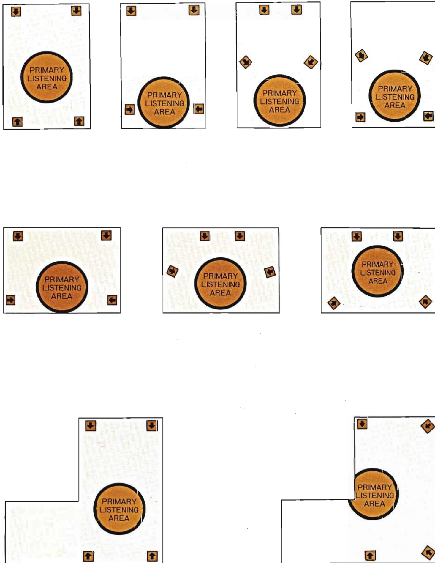
Figure 3. Disposition des haut-parleurs.
