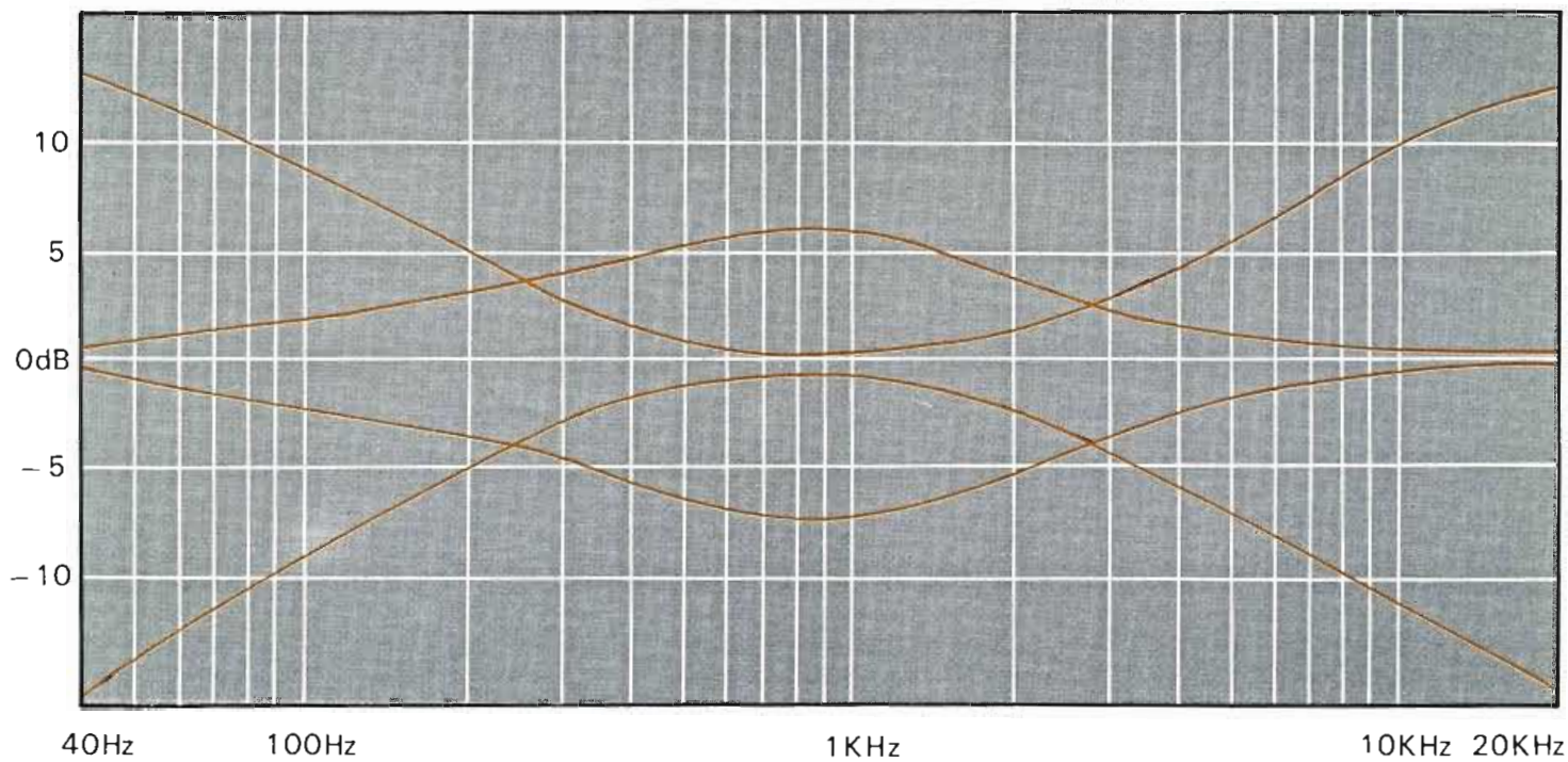
Figure 7. Caractéristiques des contrôles de tonalité
