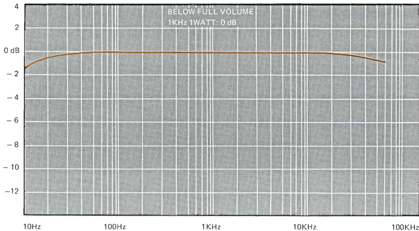
Figure 11. Réponse en fréquences
