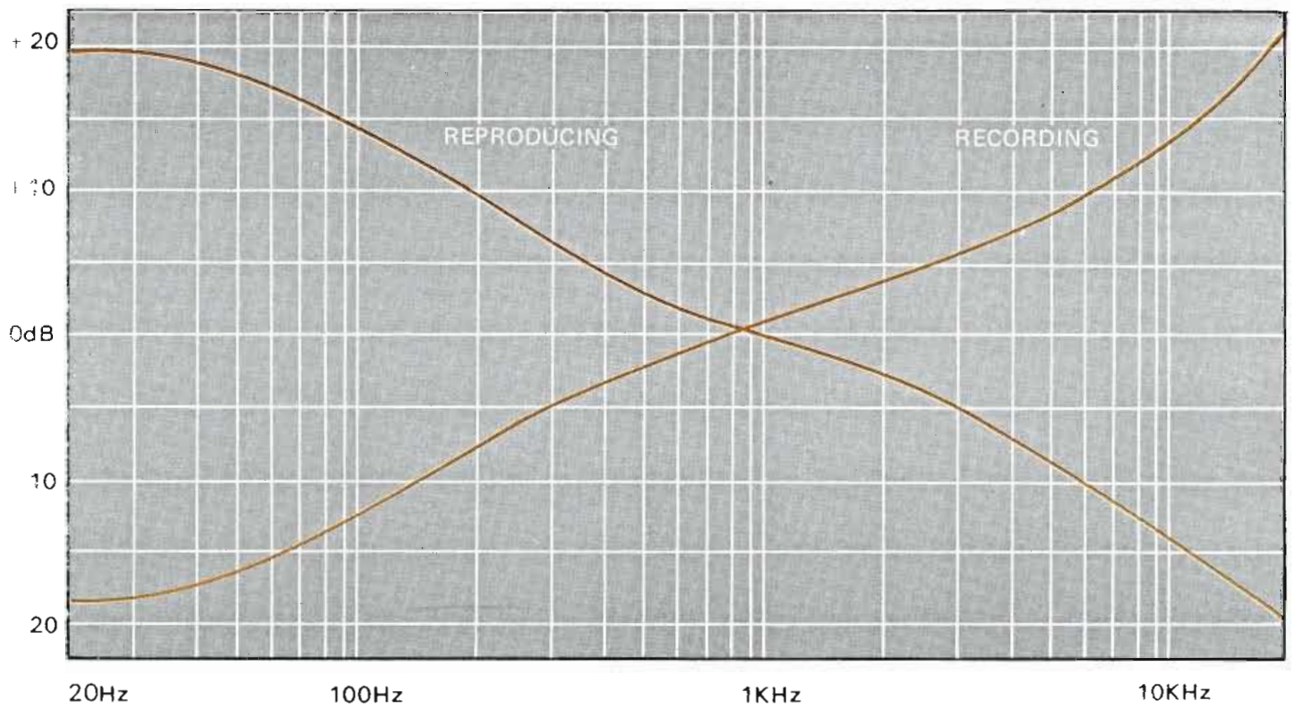
Figure 9. Caractéristiques du réseau correcteur phonographique
